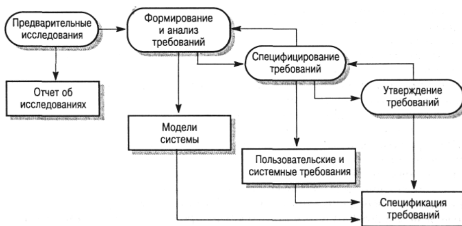
Рис.12.1. Порядок формирования требований к информационной системе
