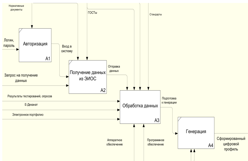
Рис. 3.1. Диаграмма декомпозиции первого уровня в нотации IDEF0
