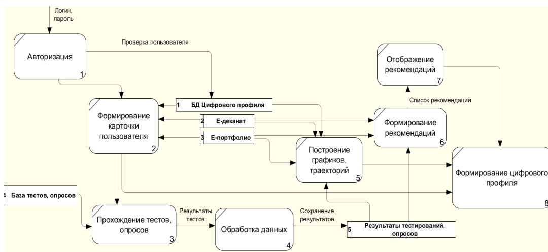
Рис.5.3. Диаграмма потоков данных «Цифровой профиль»
