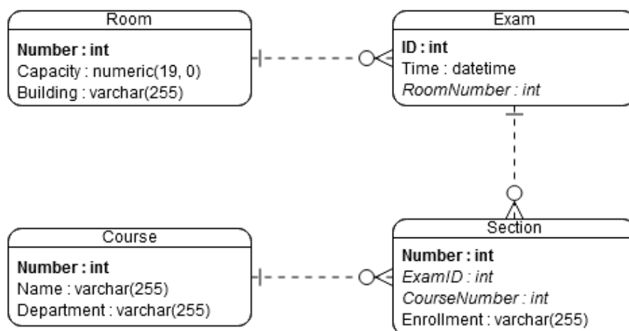
Рис. 10.1. ER-диаграмма системы планирования экзаменов
