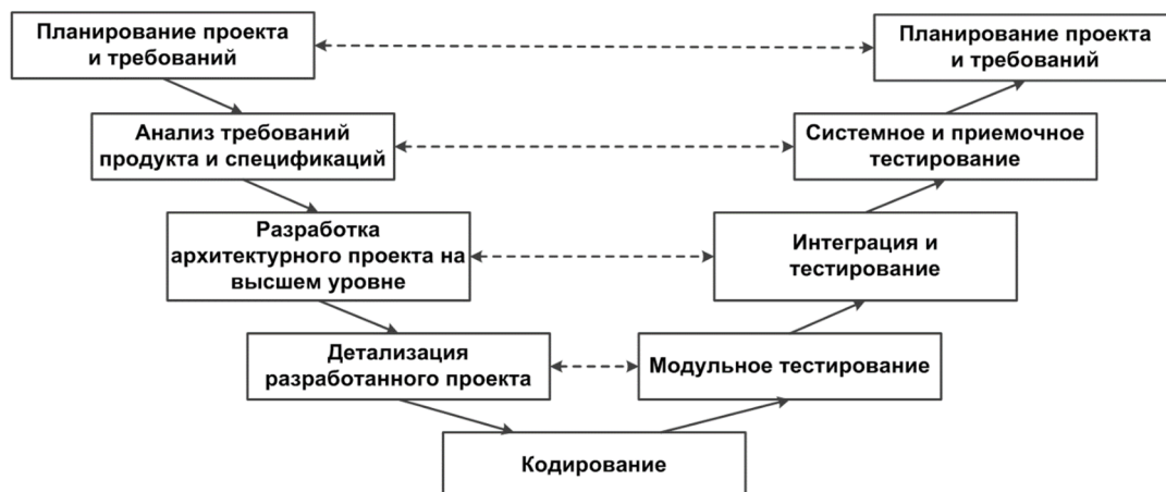
Рис. 8.2. V-модель процесса разработки программного обеспечения
