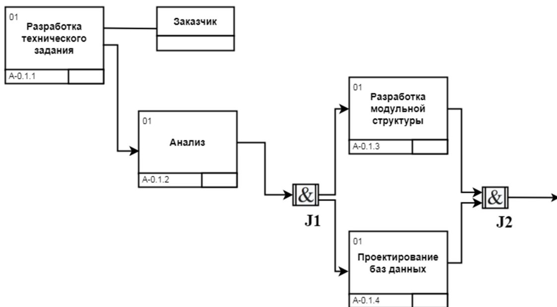
Рис. 6.1. Контекстная диаграмма «Разработка системы службы занятости»
