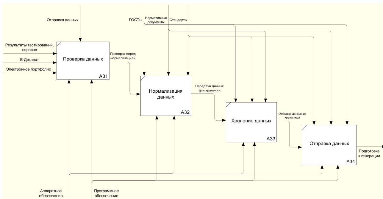
Рис. 4.2. Декомпозиция второго уровня модели нотации IDEF0
