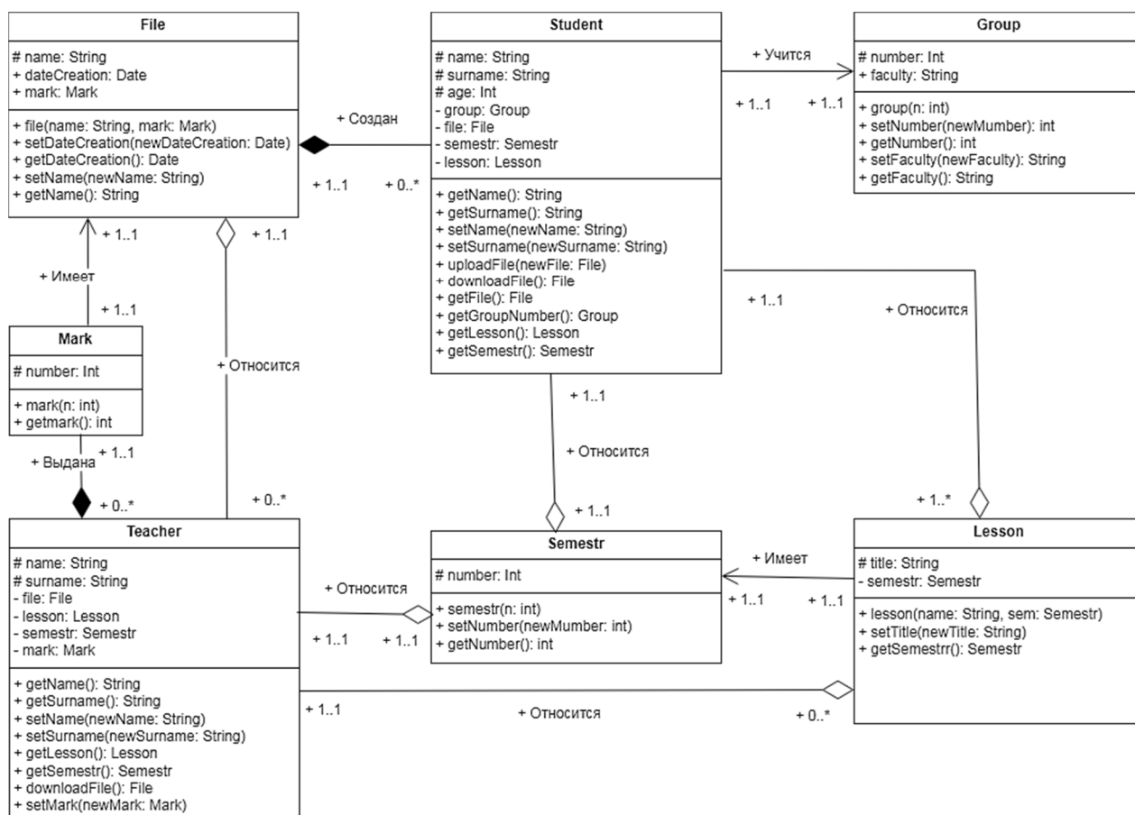
Рис. 7.5. Пример диаграммы классов
