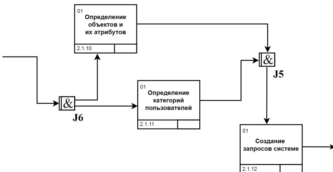
Рис. 6.2. Диаграмма декомпозиции работы «Анализ»
