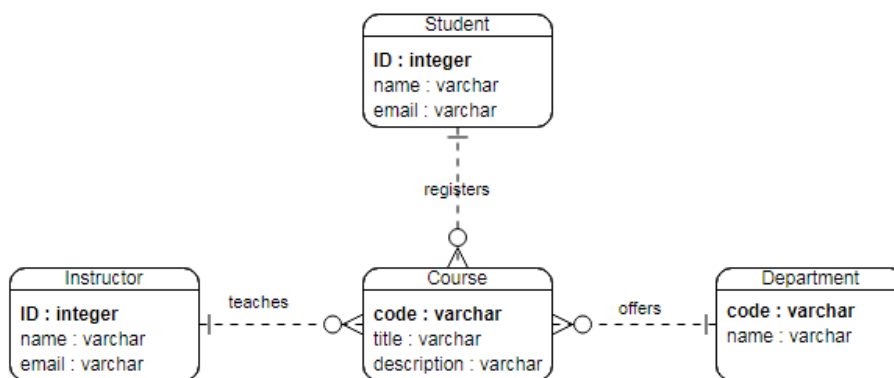
Рис. 10.2. Логическая модель данных
