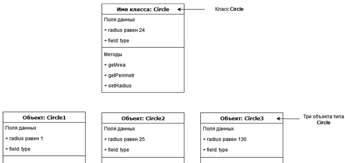
Рис. 7.1. Пример диаграммы класса Circle
