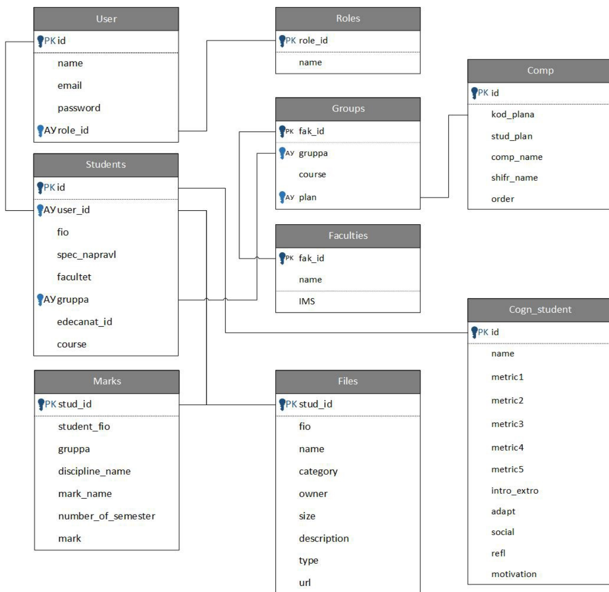
Рис. 10.2. Структура базы данных для веб-приложения «Цифровой профиль»
