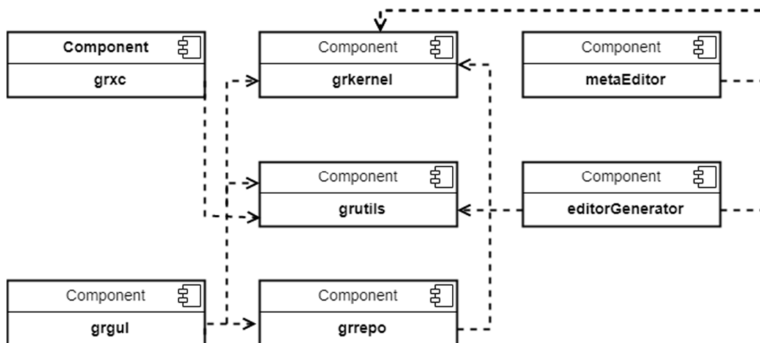
Рис. 9.1. Диаграмма компонентов программной системы
