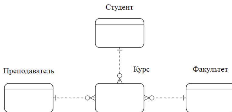
Рис. 10.1. Концептуальная модель данных
