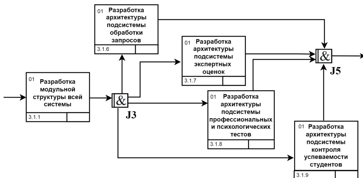
Рис. 6.3. Диаграмма декомпозиции работы «Разработка модульной структуры»
