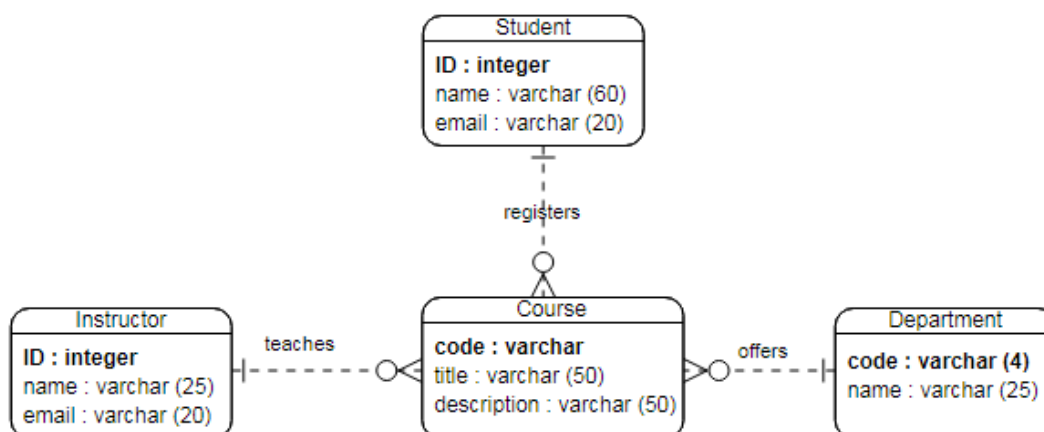
Рис. 10.3. Физическая модель данных
