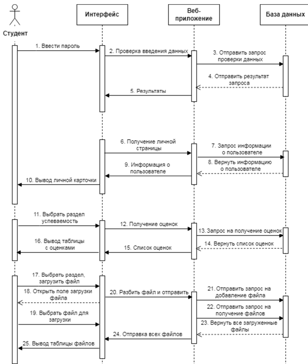
Рис. 7.4. Пример диаграммы последовательностей
