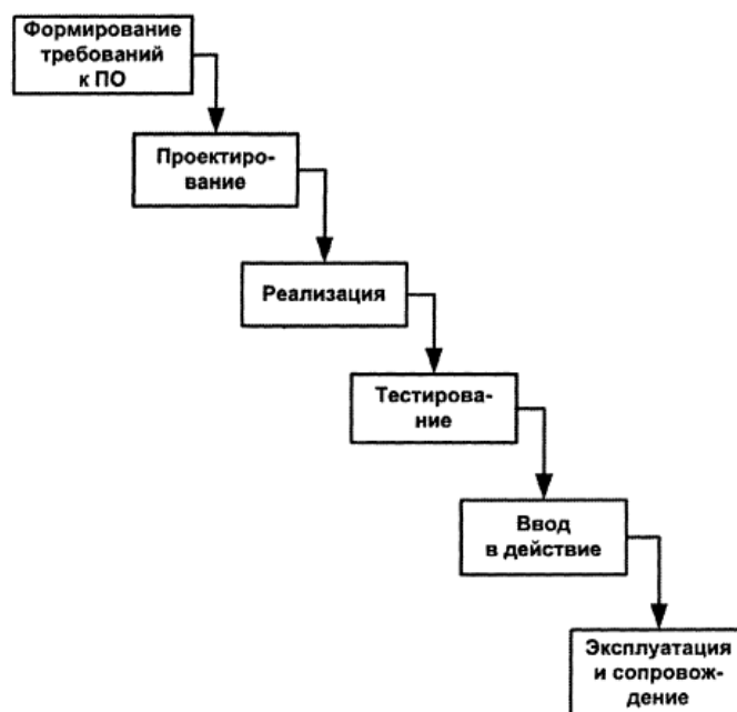
Рис. 8.1. Каскадная модель
