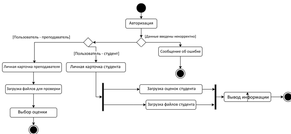
Рис. 7.6. Диаграмма состояний при работе пользователей в системе электронного портфолио
