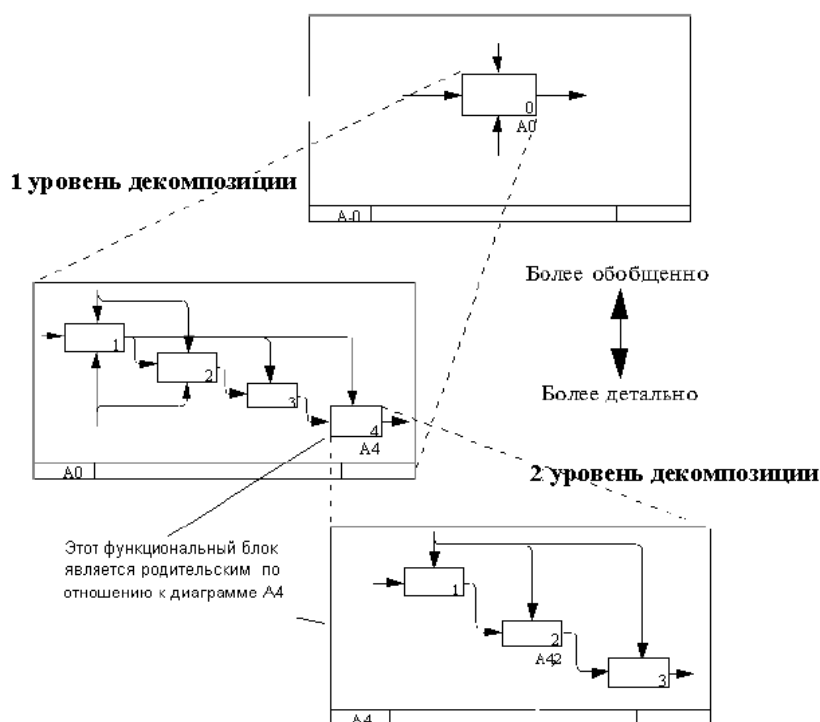
Рис. 4.1. Декомпозиция функциональных блоков первого и второго уровня
